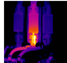
Fehlerhafte Sicherung
